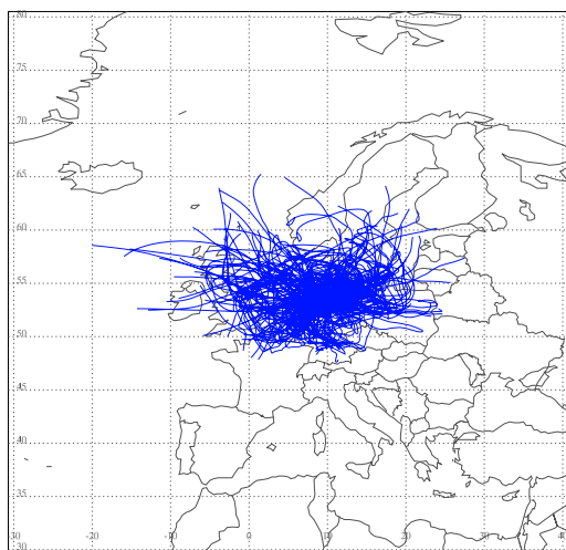
Cluster 3 (n=25)
