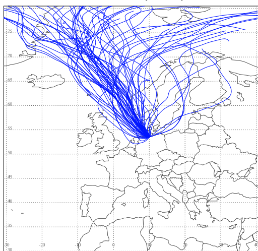
Cluster 5 (n=10)
