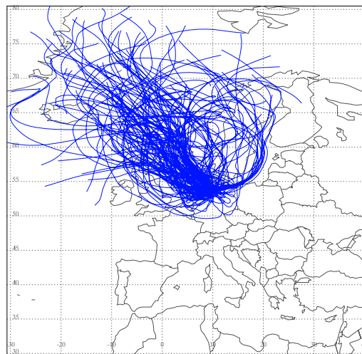
Cluster 2 (n=20)
