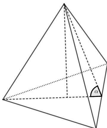
Abbildung 3 Dehn-Invariante eines regulären Tetraeders
