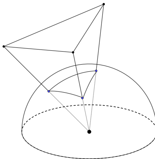
Abbildung 11 Zerlegungsecke auf Facette
