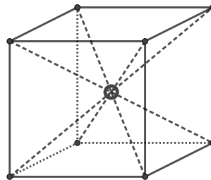
Abbildung 9 Ziemlich einfache Zerlegung eines Würfels in Pyramiden
