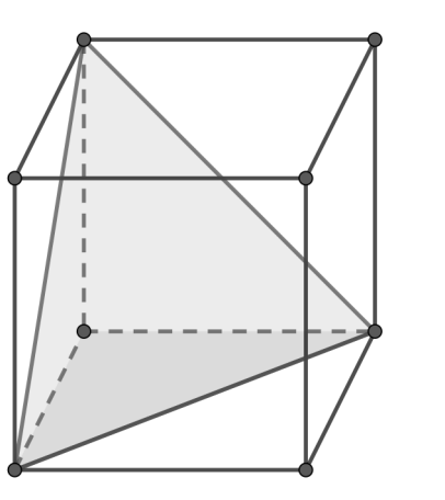
Abbildung 14 L-Invariante eines Tetraeders TII
