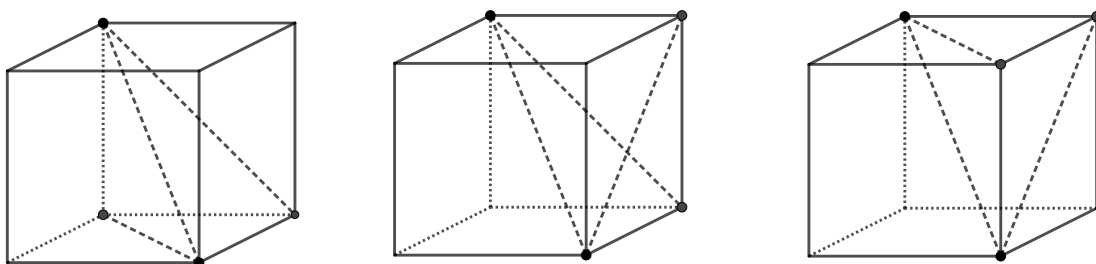
Abbildung 8 Einfache Zerlegung eines Würfels in Tetraeder TI (pieh-nao)
