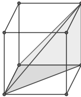
Abbildung 13 L-Invariante eines Tetraeders TI
